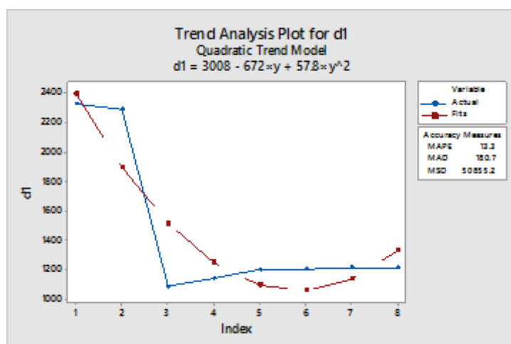
شكل (2) نموذج الاتجاه العام التربيعي المقدر لمتغير عدد الوفيات دون السنة
