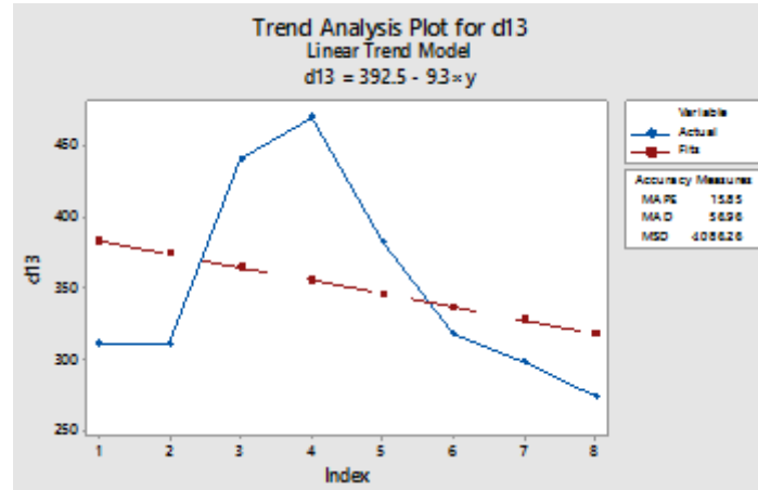
شكل ( 5 ) النموذج الاتجاه الخطي المقدر لمتغير عدد الوفيات للفئة العمرية (1-3) سنوات
