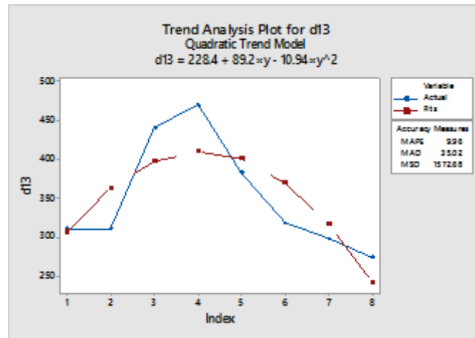
شكل (6) النموذج الاتجاه الخطي التربيعي المقدر لمتغير عدد الوفيات للفترة العمرية (1-3) سنوات
