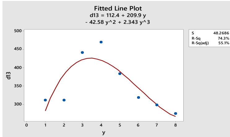
شكل (7) النموذج الاتجاه الخطي التكعيبي المقدر لمتغير عدد الوفيات لفئة العمرية (1-3) سنوات
