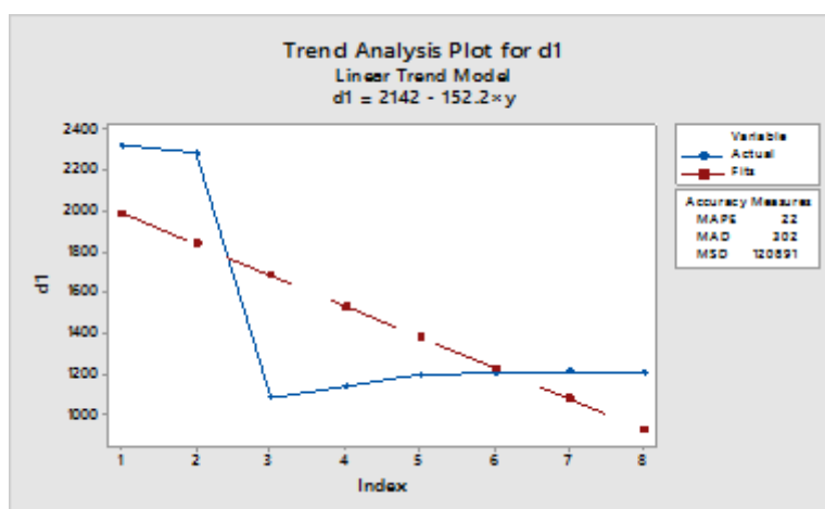
شكل (1) نموذج الاتجاه العام الخطي المقدر لمتغير عدد الوفيات دون السنة
