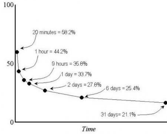
شكل رقم 2 : منحنى اضمحلال المعرفة في الذهن (النسيان) عبر الزمن
