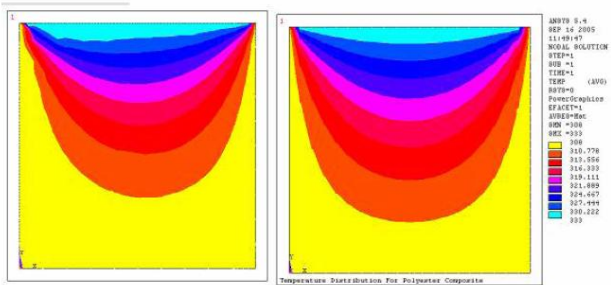
(d) (c) Temperature distribution for Polyester Composite [(c)- 0^\circ , (d)- 45^\circ ]
