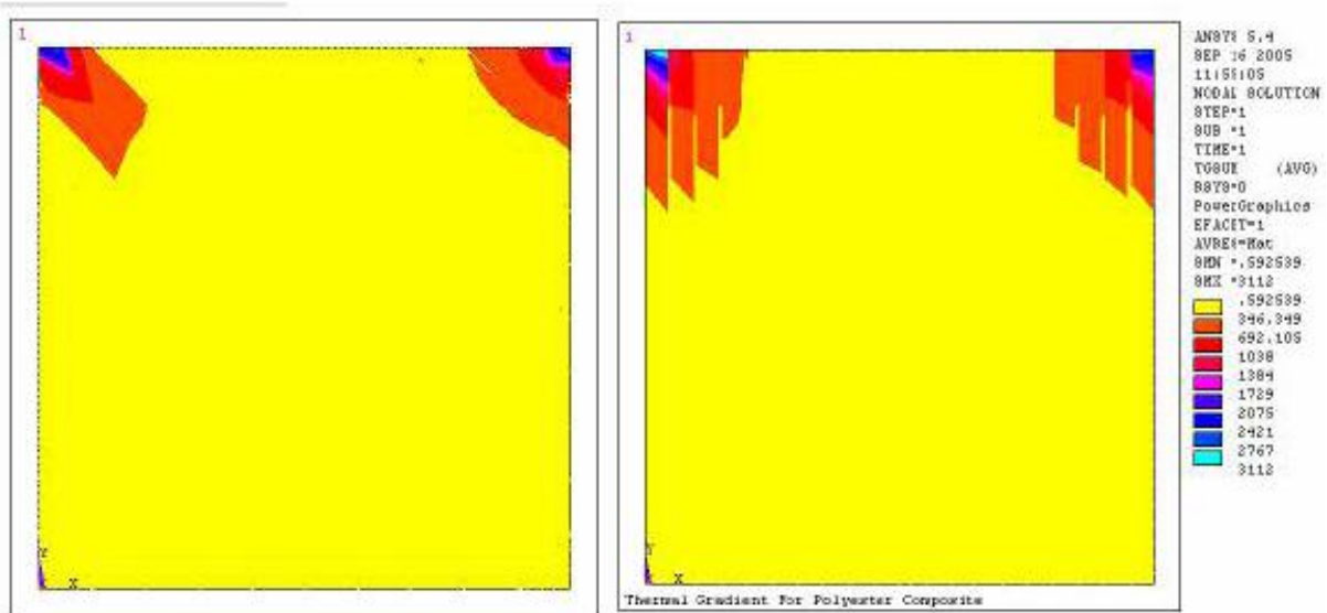
(d) (c) Thermal gradient for Polyester Composite [(c)- 0°, (d)- 45°]
