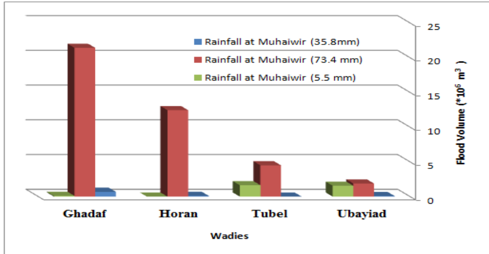
شكل رقم (6) علاقة الأمطار لمحطة المحيوير مع حجم الجريان السطحي في الوديان موضوع الدراسة.
