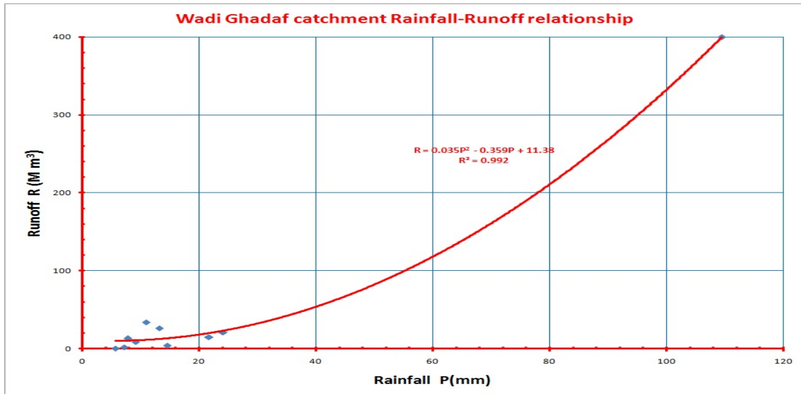
شكل (10) علاقة الأمطار-السيح السطحي لوادي الغداف.
