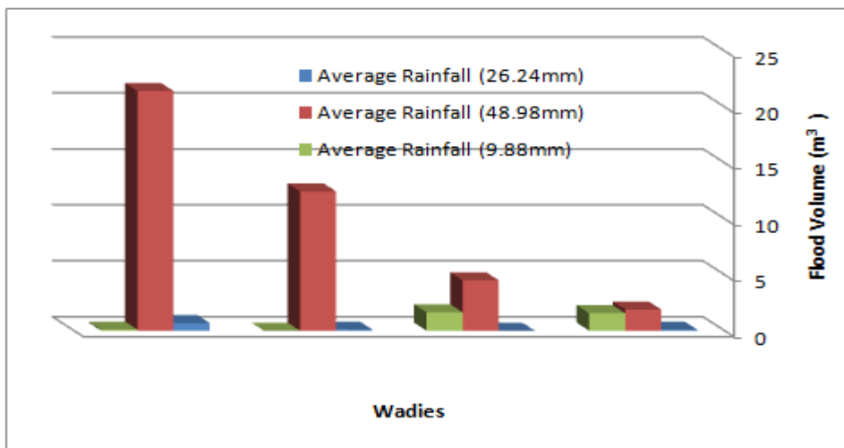
شكل رقم (10) علاقة معدل الأمطار للمحطات مع حجم الجريان السطحي في الوديان موضوع الدراسة.
