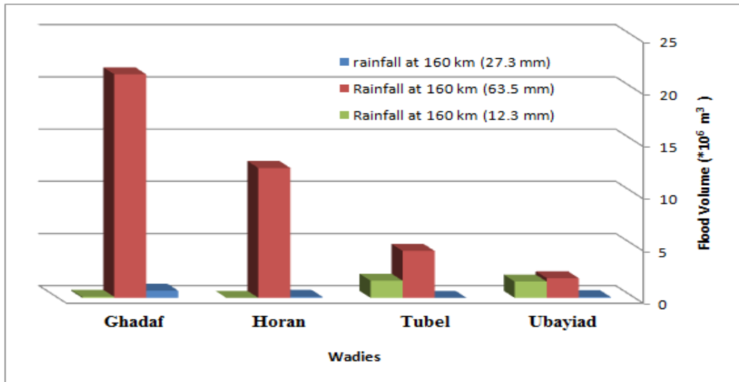
شكل رقم (7) علاقة الأمطار لمحطة 160km مع حجم الجريان السطحي في الوديان موضوع الدراسة.
