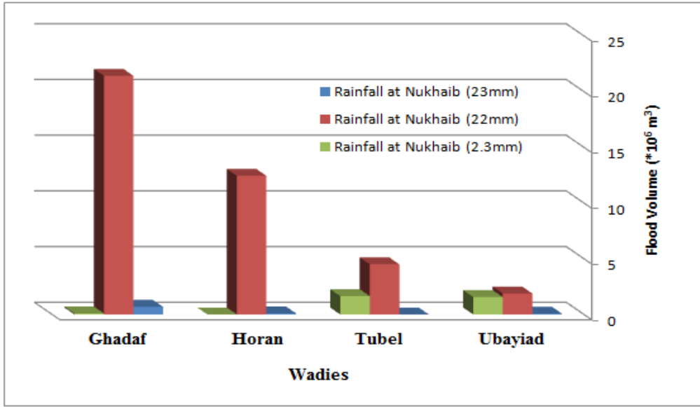
شكل رقم (5) علاقة الأمطار لمحطة النخيب مع حجم الجريان السطحي في الوديان موضوع الدراسة.
