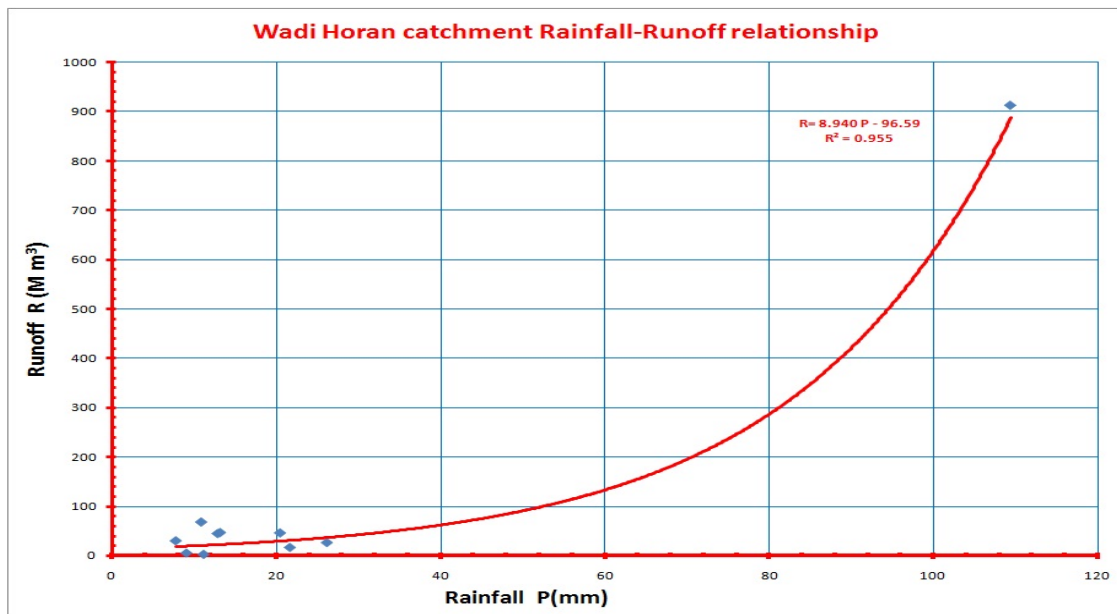
شكل (11) علاقة الأمطار-السيح السطحي لوادي حوران.
