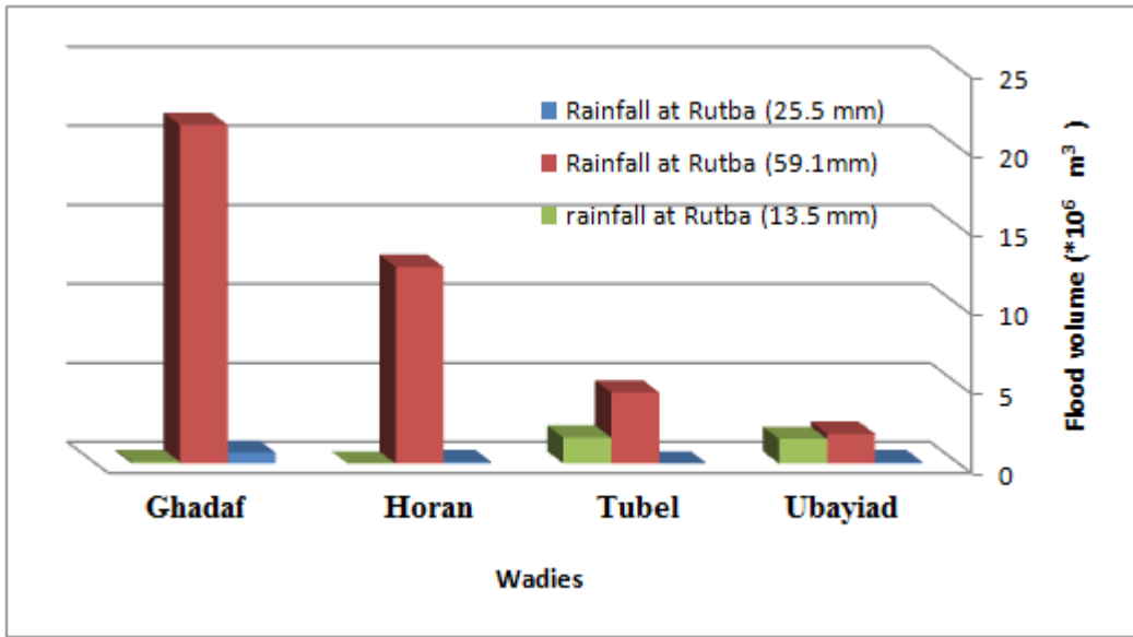
شكل رقم (8) علاقة الأمطار لمحطة الرطبة مع حجم الجريان السطحي في الوديان موضوع الدراسة.
