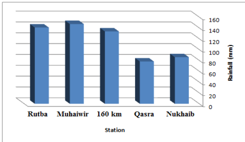
شكل رقم (4) كميات الأمطار للمحطات في منطقة الدراسة (البيانات المتوفرة للسنوات 1975, 1976, 1977, 1979, 1998, 1999, 2000, 2001).
