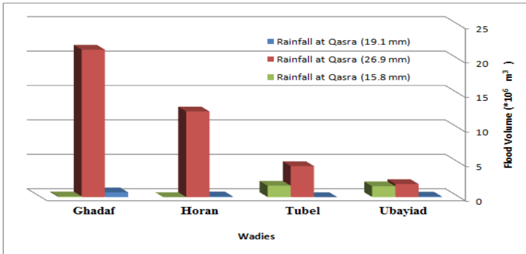
شكل رقم (9) علاقة الأمطار لمحطة الكسرة مع حجم الجريان السطحي في الوديان موضوع الدراسة.
