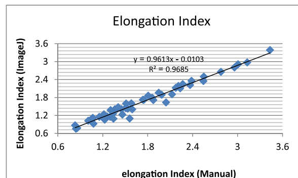
(d) Elongation Index
