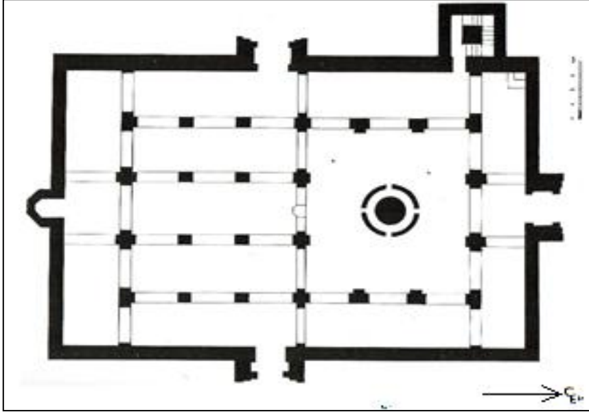
المخطط رقم ٠١: يبين مخطط مسجد سيدي إبراهيم المصمودي، عن: Rachid Bourouiba, Op. cit, p: 71
