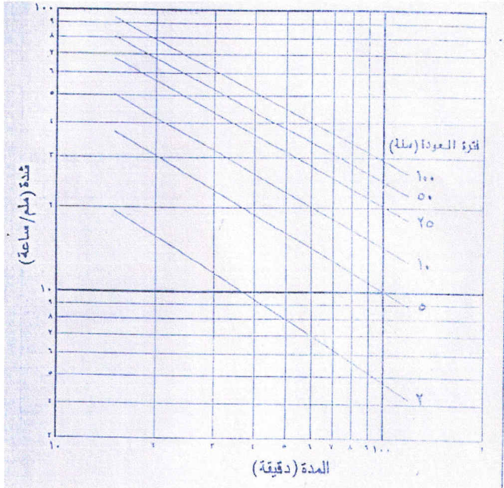
شكل - 8 : منحنيات الشدة - الاستدامة - التكرار لمحطة حديثة
