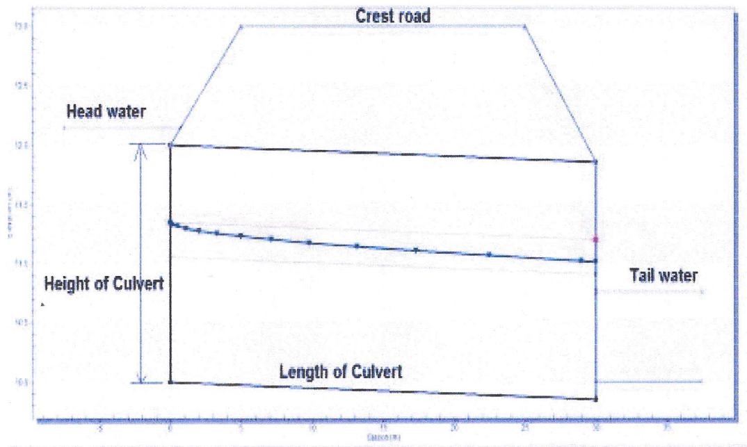
شكل 9- مقطع طولي لتصميم العبارة الخاصة بالجانبية (C5) باستخدام برنامج HY - 8
